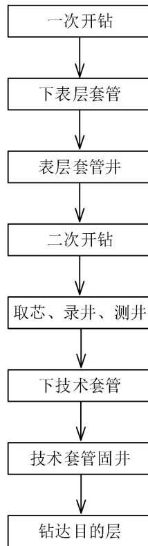
图 2-3 钻井工艺流程图
