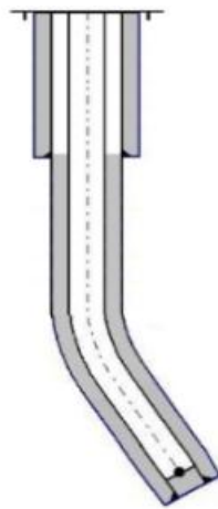
图 2-1 花 110 斜井井身结构图
