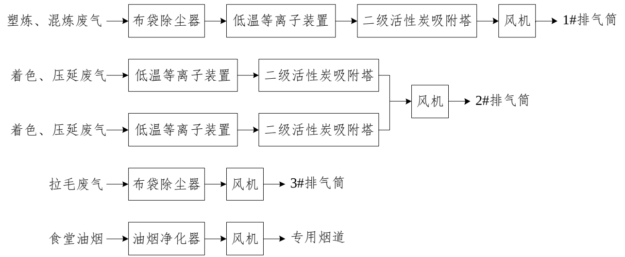
图 6.1-1 废气治理措施示意图
