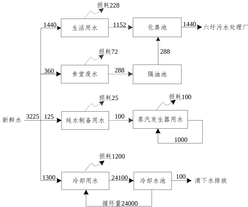
图 3.3-2 项目水平衡图 单位：m 3 /a
