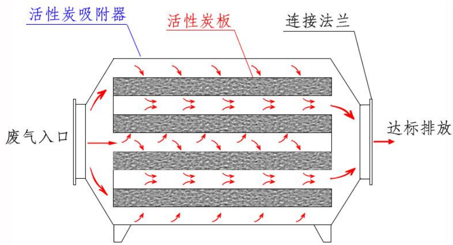
图 6.1-3 活性炭吸附装置工作原理图
