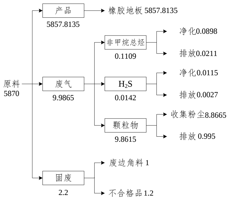
图 3.3-1 项目总体工程物料平衡图 单位：t/a
